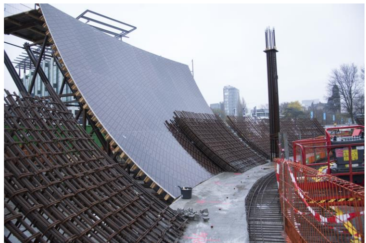
Eerste buitenbekisting
